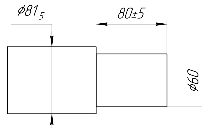
Рекомендованный посадочный кронштейн
